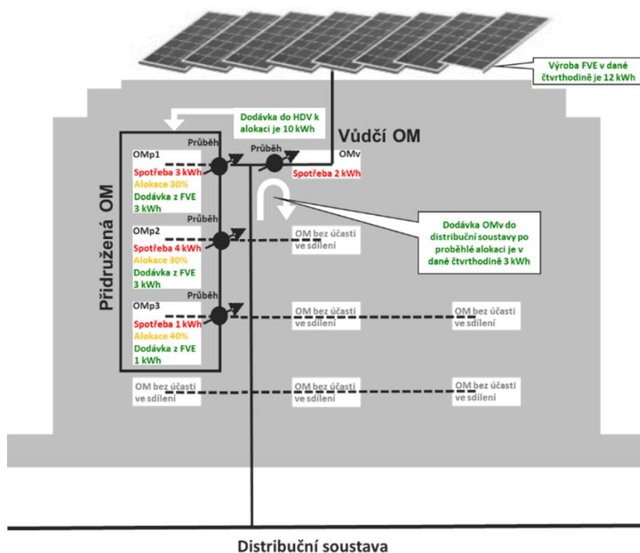
Obrázek 30: Schéma výroby elektřiny v bytovém domě a její rozdělení mezi jednotky
