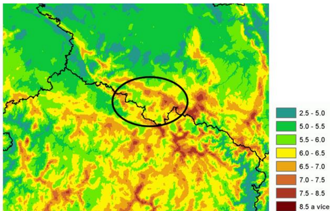
Obrázek 26: Větrná mapa ČR 100 metrů nad povrchem
