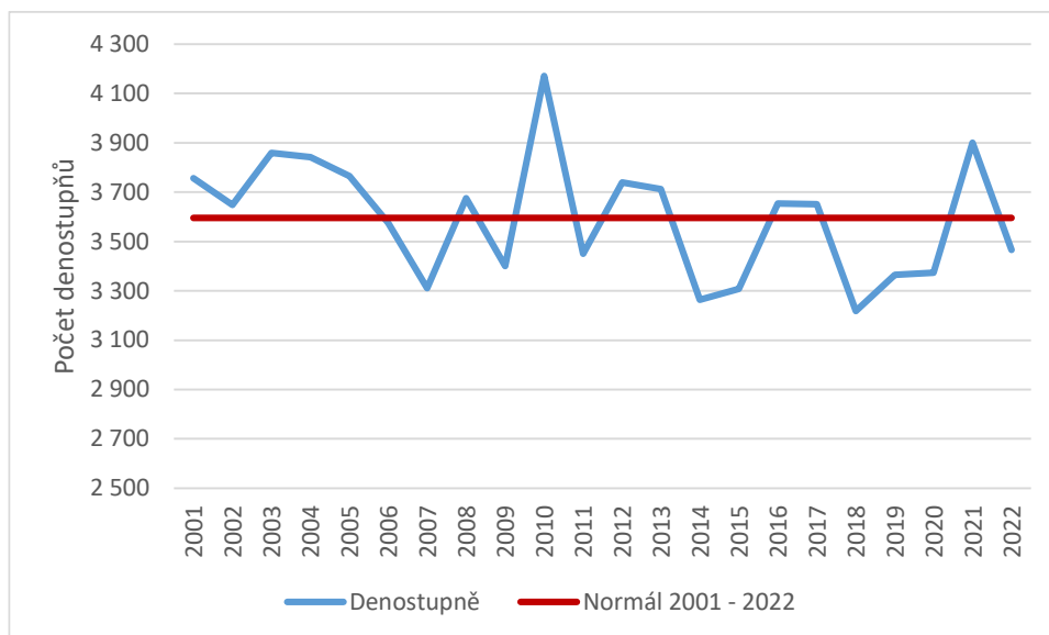
Obrázek 17: Průběh denostupňů pro meteorologickou stanici Pardubice
