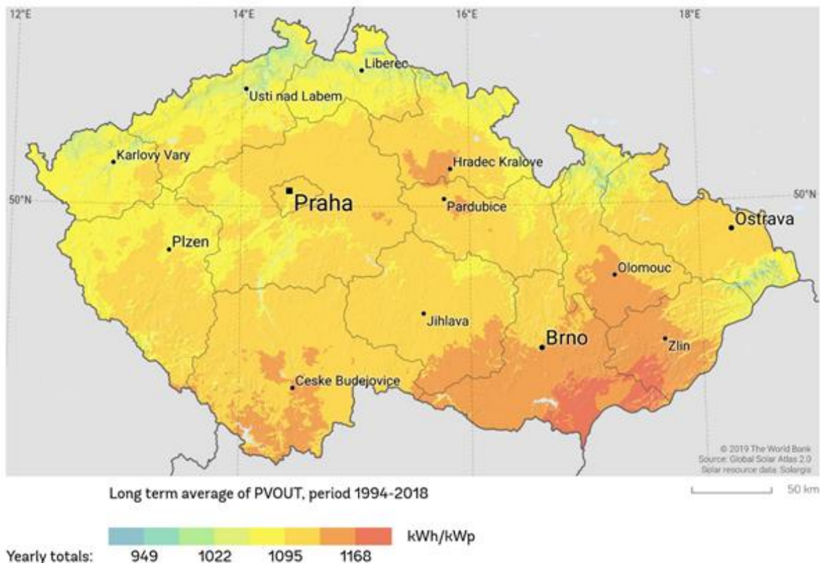
Obrázek 7: Mapa potenciálu výroby z fotovoltaiky v ČR
