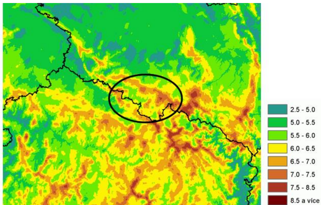
Obrázek 10: Větrná mapa ČR 100 metrů nad povrchem
